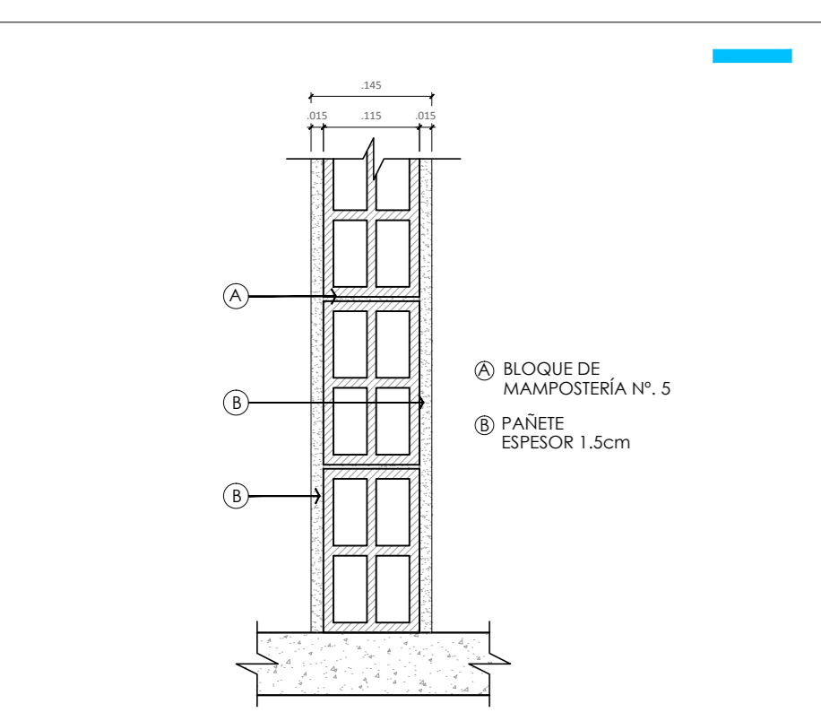
DETALLE DE ESPECIFICACIONES MURO STC 42 ALTERNATIVA CONSTRUCCIÓN MAMPOSTERÍA
