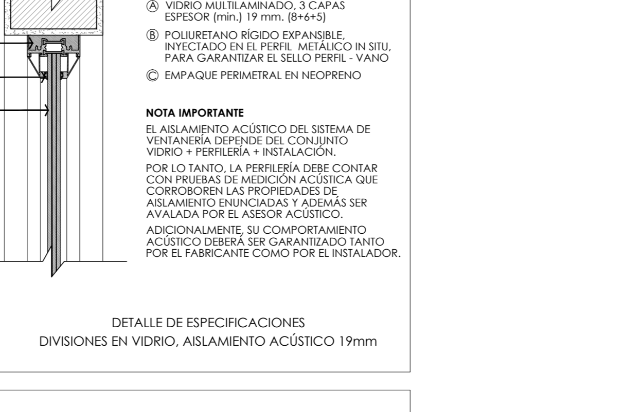
DETALLE DE ESPECIFICACIONES DIVISIONES EN VIDRIO, AISLAMIENTO ACÚSTICO 19mm
