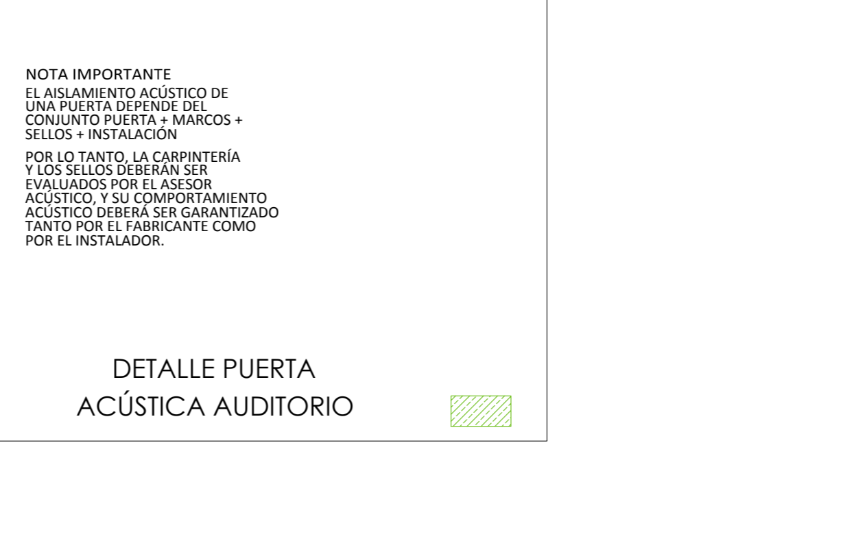
DETALLE PUERTA ACÚSTICA AUDITORIO
