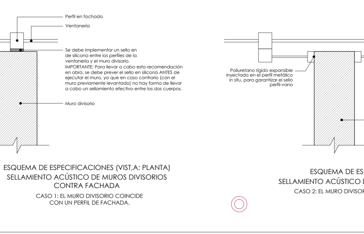
ESQUEMA DE ESPECIFICACIONES (VISTA: PLANTA) SELLAMIENTO ACÚSTICO DE MUROS DIVISORIOS CONTRA FACHADA
